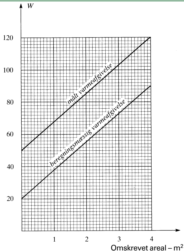
Figur 6.1 – Tilladelig varmeafgivelse fra mindre varmevekslere, varmtvandsbeholdere, vandvarmere og lignende som funktion af det omskrevne areal
