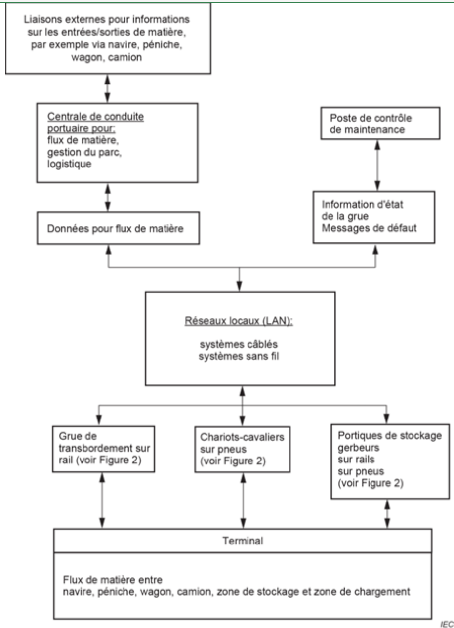
Figure 1 – Schéma fonctionnel d'appareils de levage associés dans un système type de manutention portuaire
